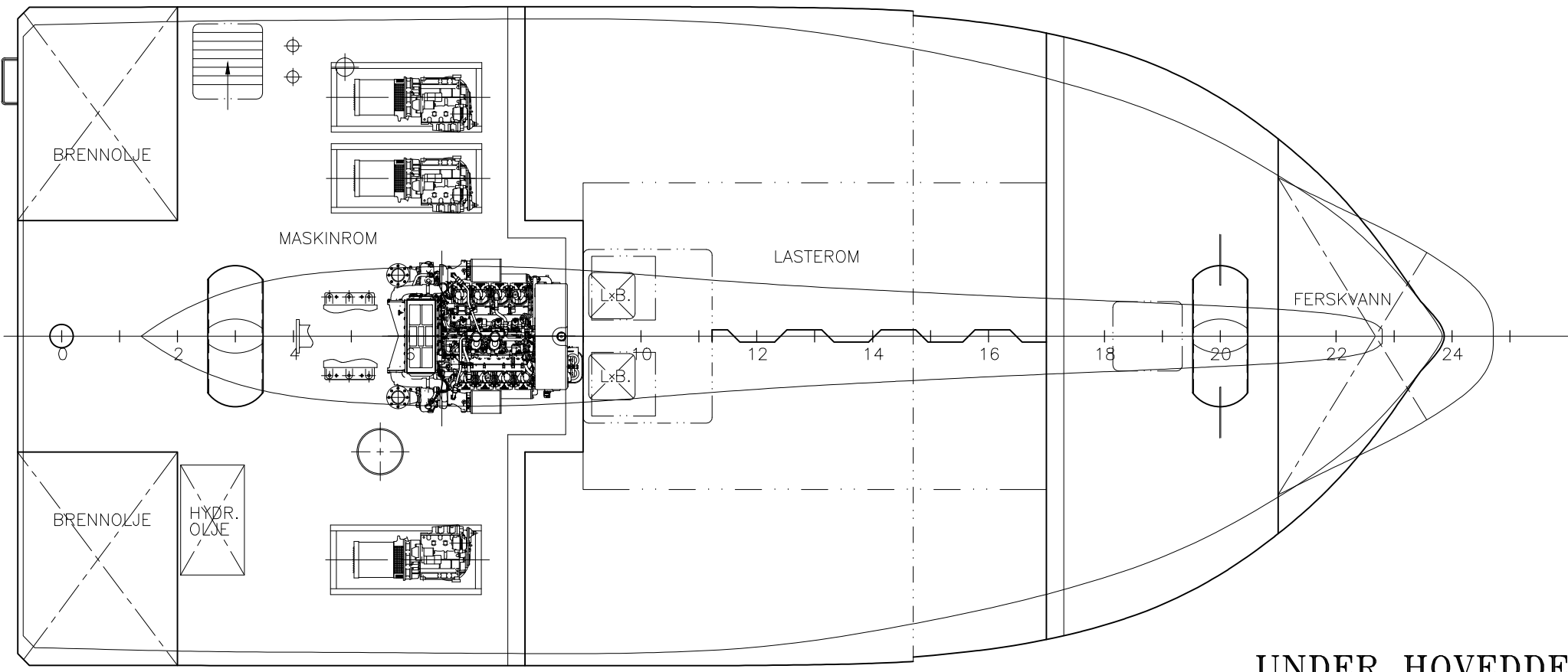
UNDER HOVEDDEKK
