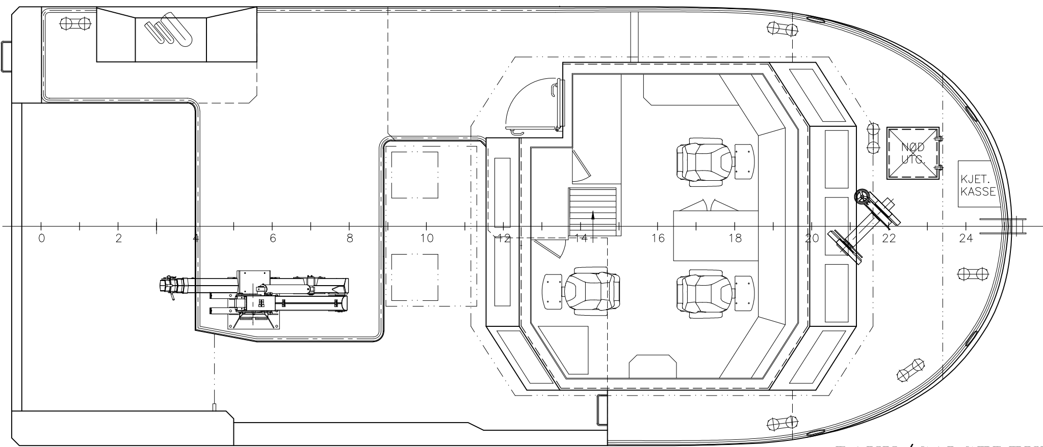
BAKK/GALGEDEKK
