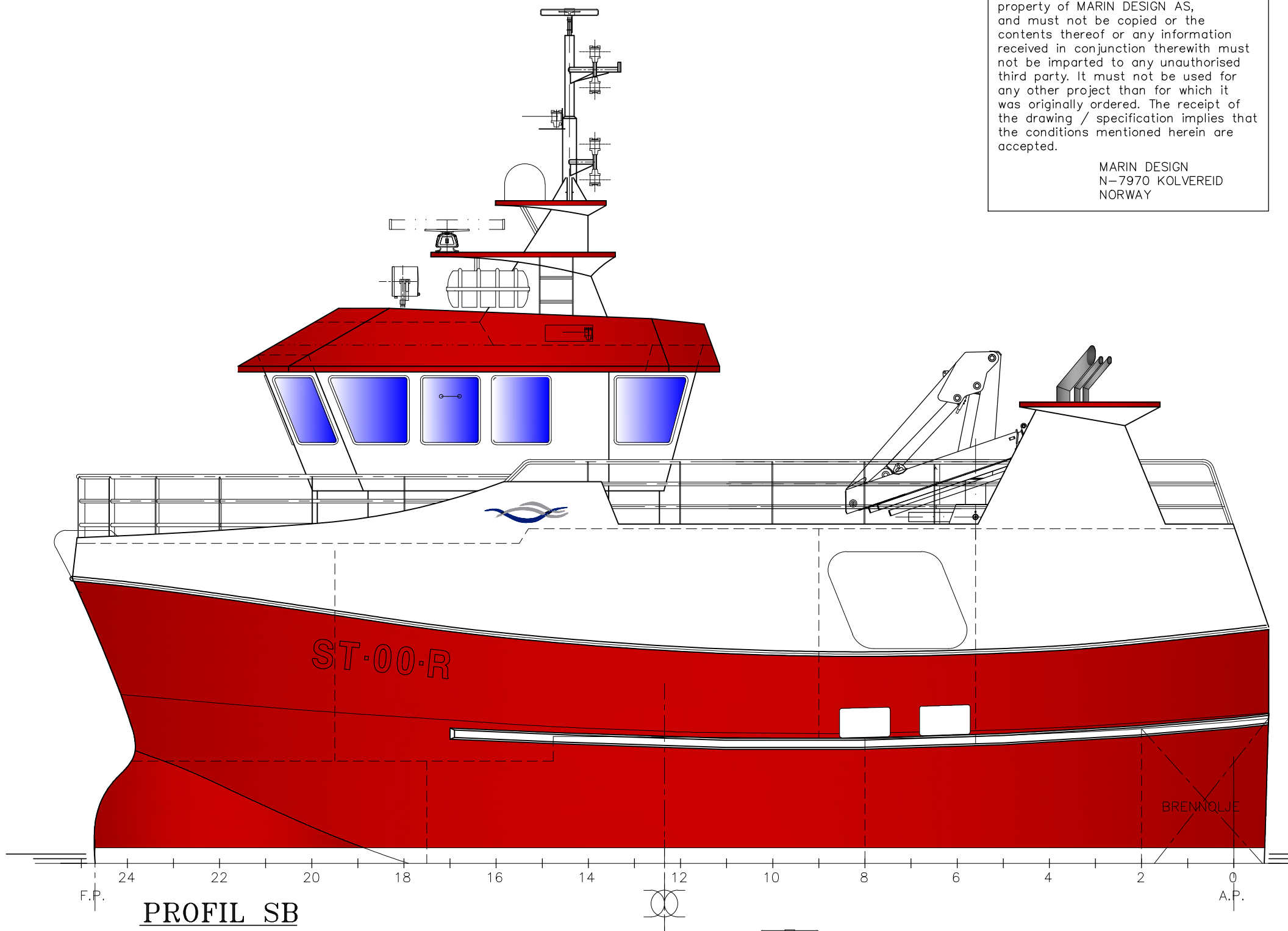
PROFIL SB
