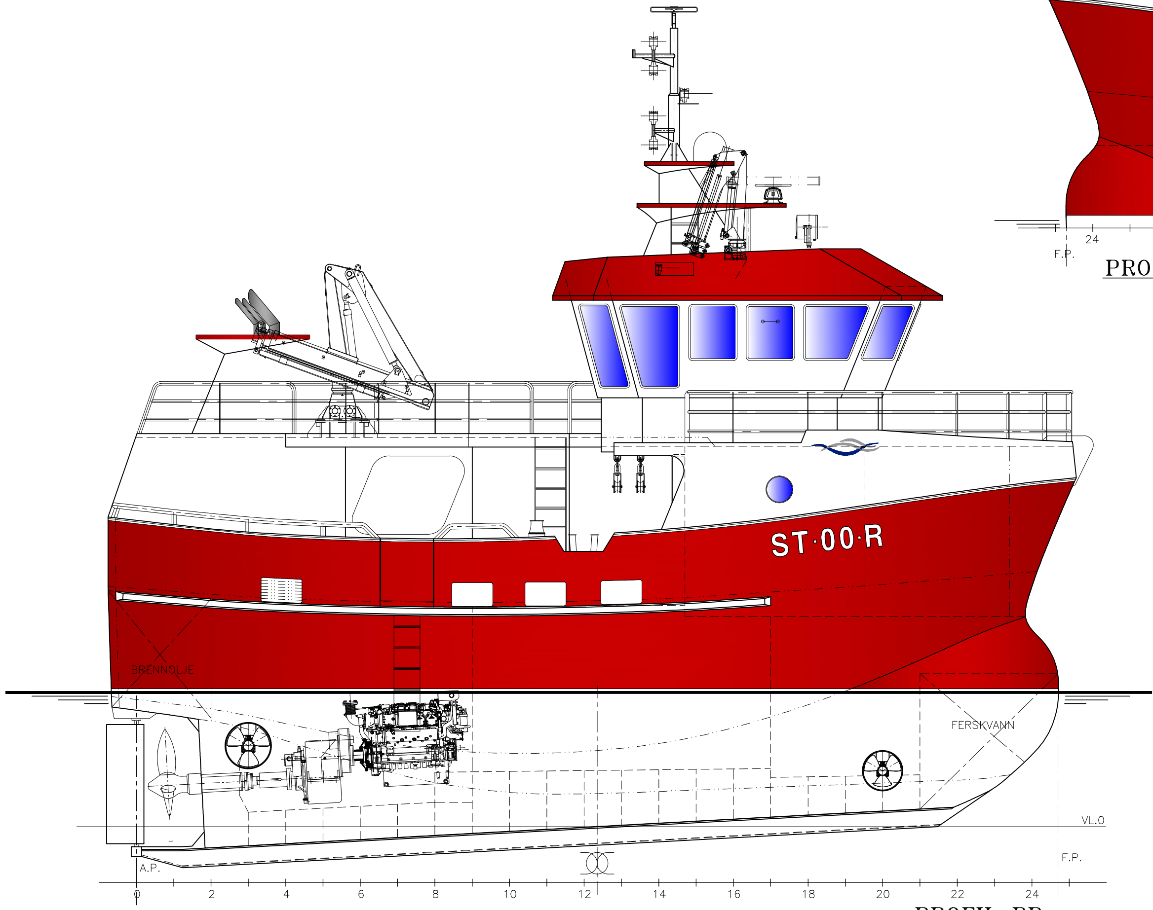
PROFIL BB
