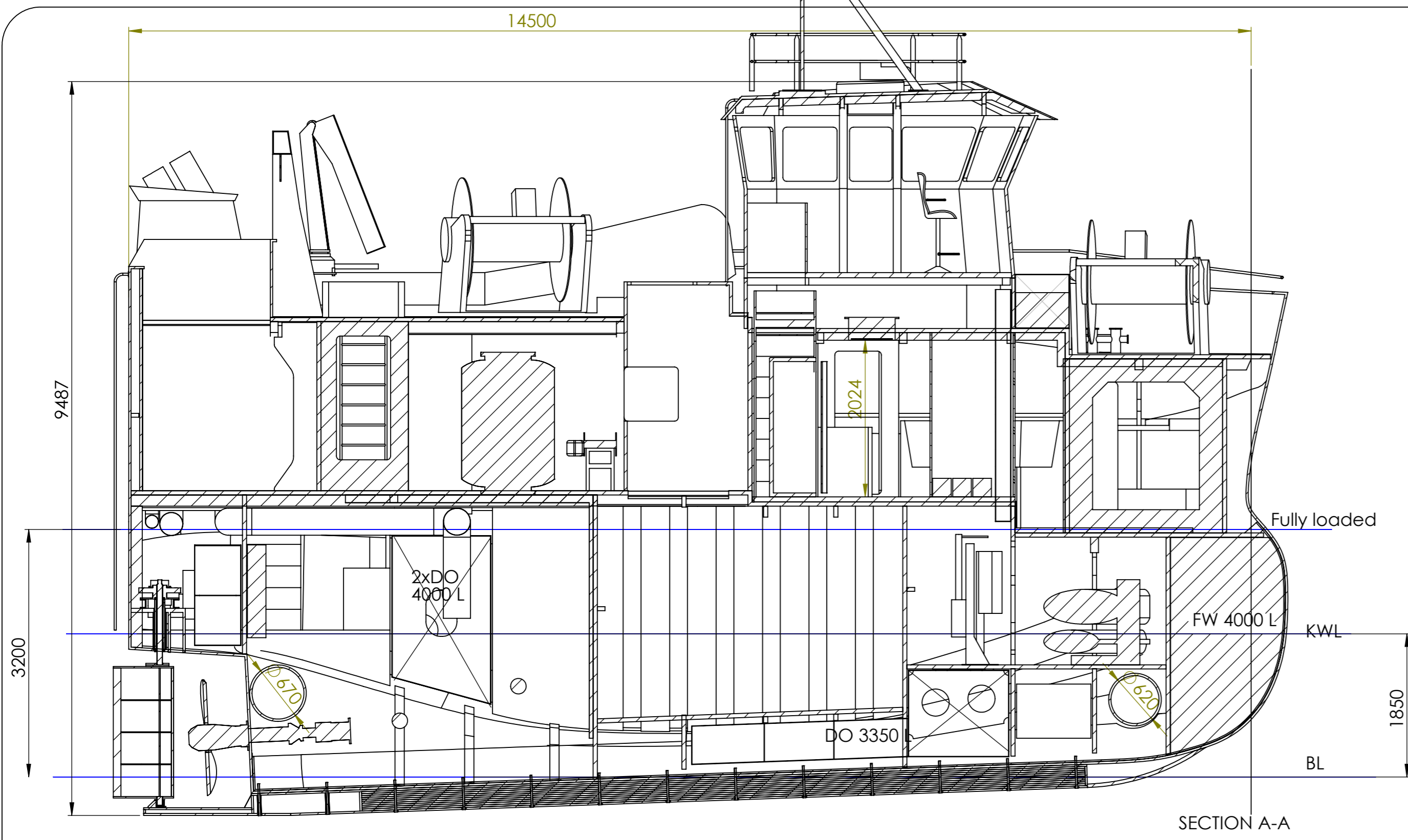
SECTION A-A
